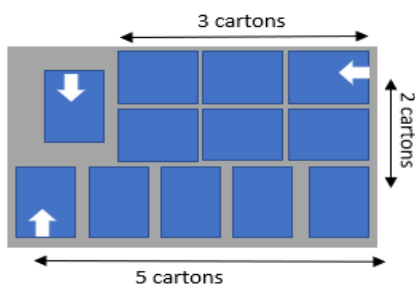
Disposition sur la palette Europe (vue du dessus) sur 5 couches
